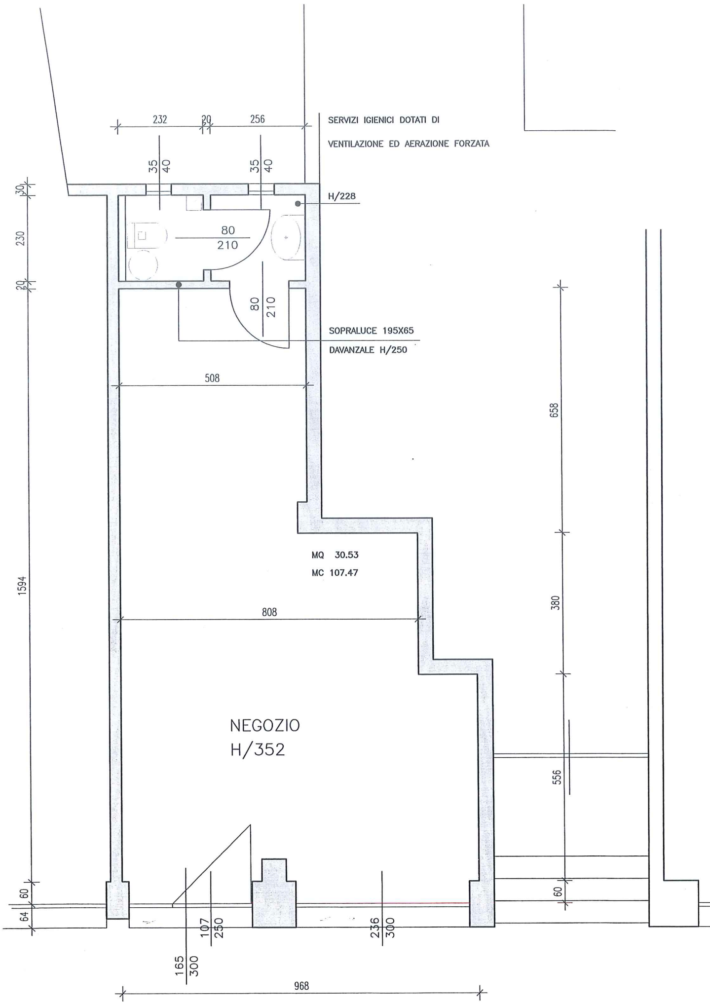
PIANTA PIANO TERRA scala disegno 1 : 50
